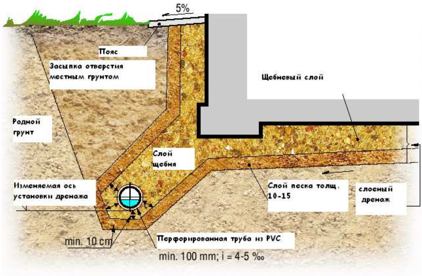
Многослойный песчано-щебневый дренаж дома в слабо пропускаемых грунтах
