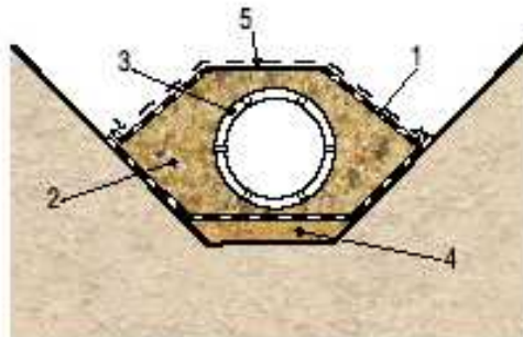
Призматический дренаж
