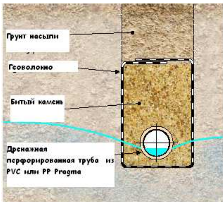
С использованием геоволокна
