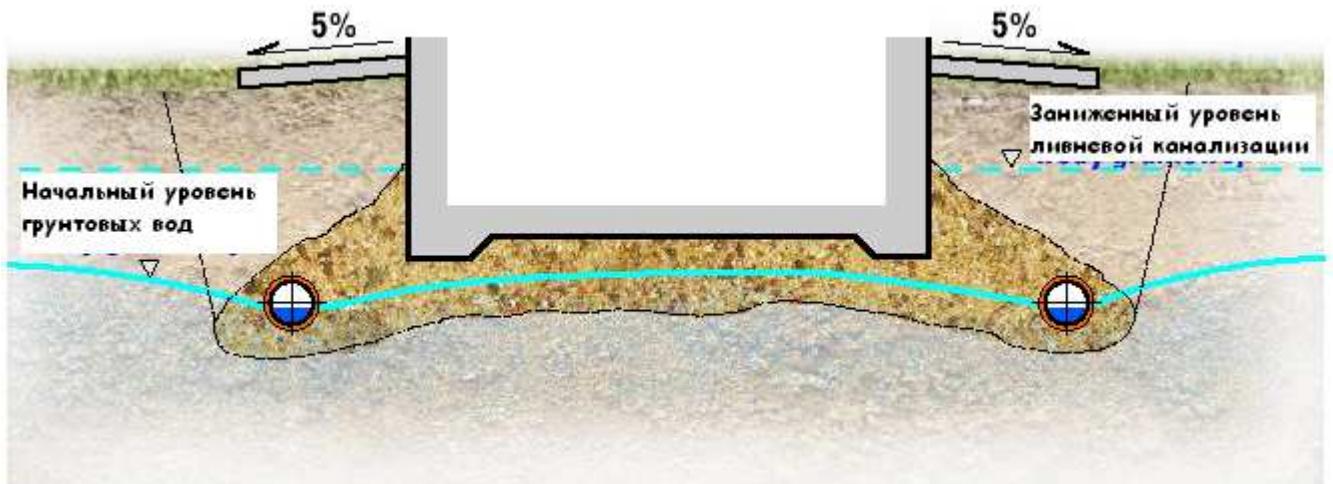
Срез дренажа дома (А-А)
