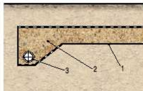
Горизонтальный слоистый дренаж
