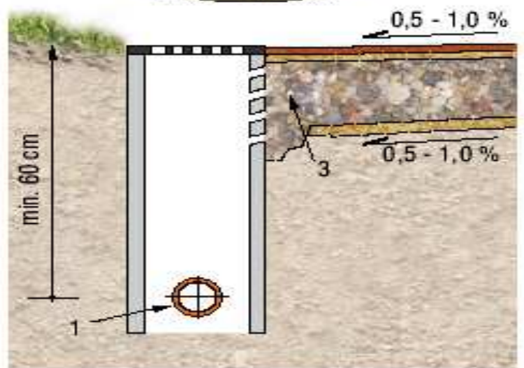
Сборный колодец, окруженный беговой дорожкой
