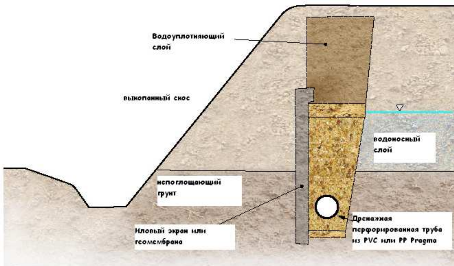
Барьерный дренаж выкопанного склона
