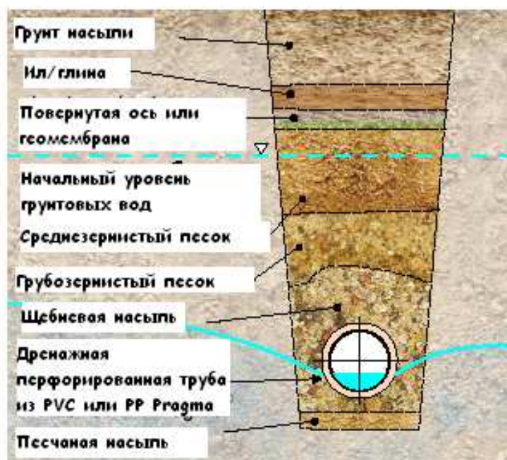
С песчано-щебневой насыпью
