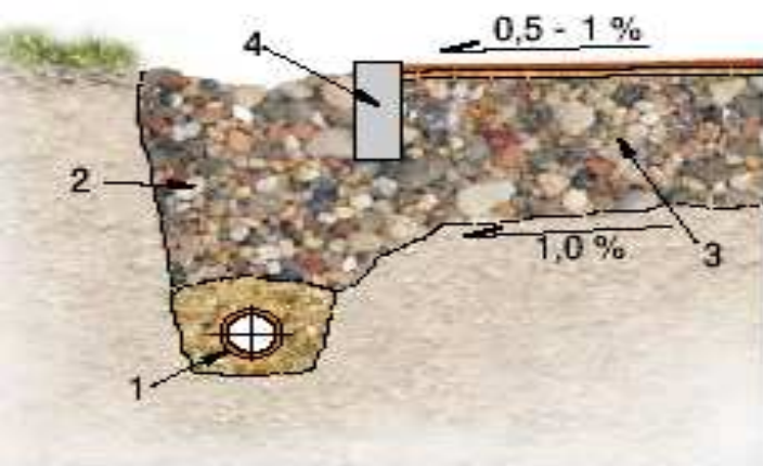
Ров, отводящий поверхностную воду с поля и беговых дорожек
