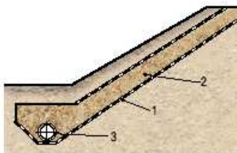
Ленточный дренаж с уклоном
